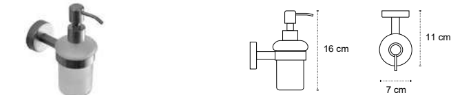
Dispenser • Distributeur de savon • Dispenser • Δοχείο υγρού σαπουνιού
